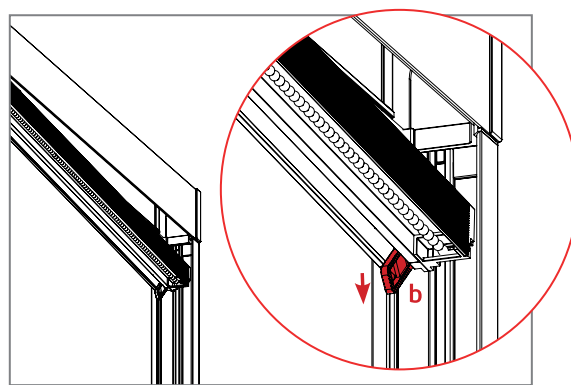
Fase 2 rimozione profilo superiore
