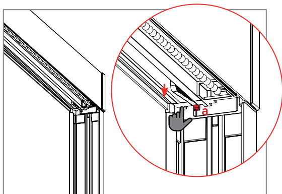
Fase 1 rimozione profilo superiore
